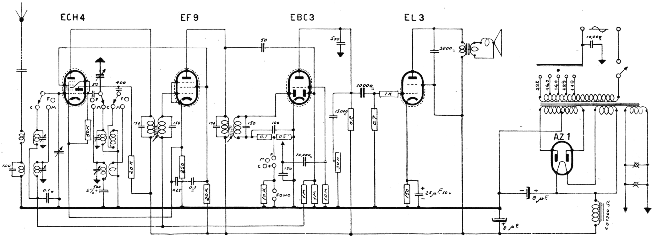
BERTONCINI RADIO - Mod. T 89. Onde medie e corte. Media frequenza: 468 kc. Bobina campo: 1200 ohm. Potenza d'uscita: 2 watt.
